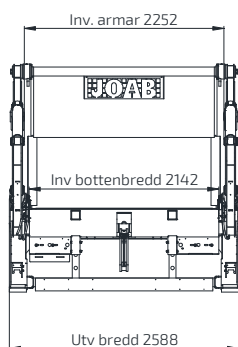
Breddmått 2600 visad (-50 för 2550 resp -100 för 2500)
